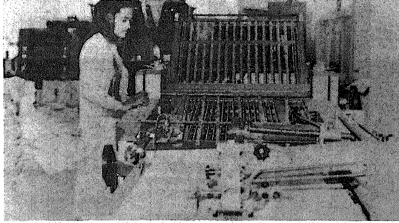
العمل بواسطة آلة التعطيف
